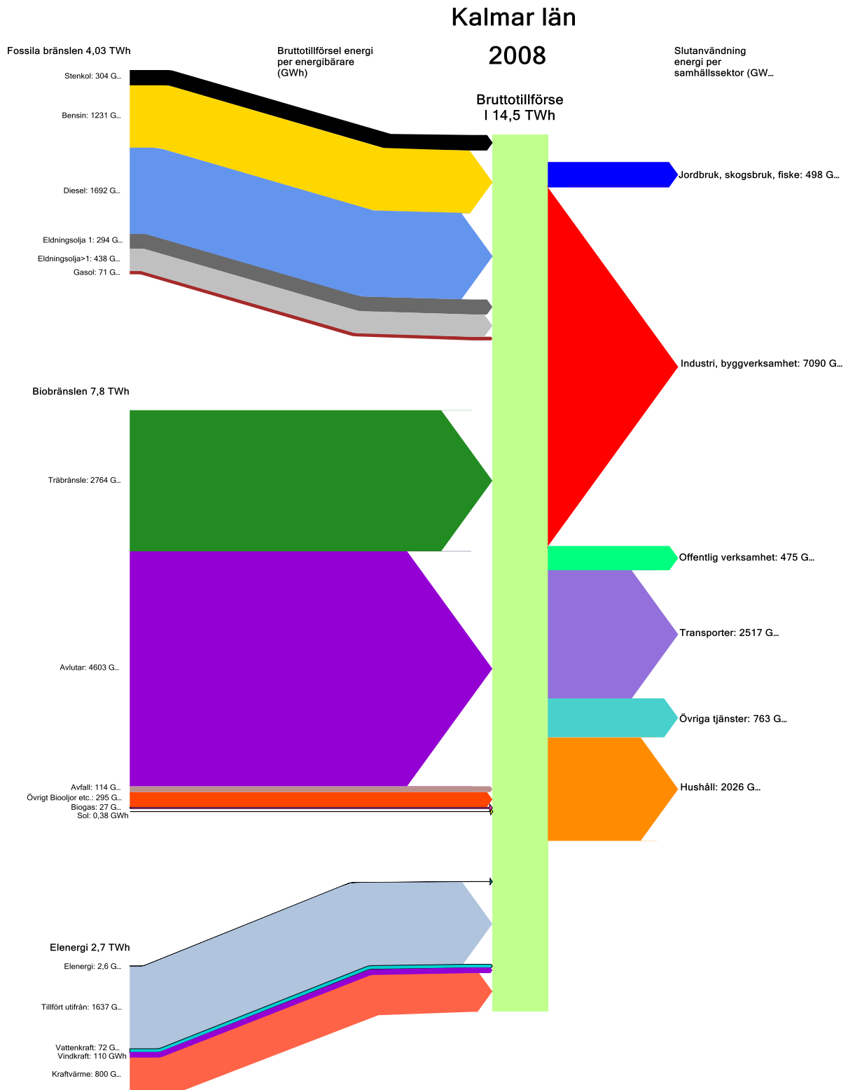
Figur 16 Sankeydiagram Energibalans Kalmar län 2008
