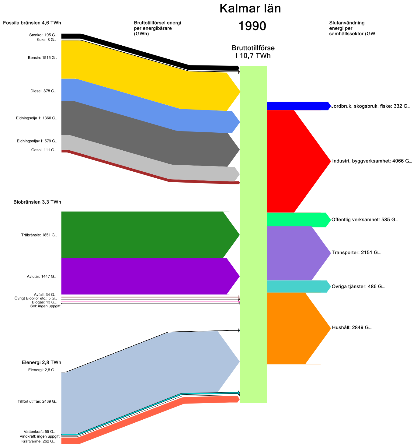
Figur 15 Sankeydiagram Energibalans Kalmar län 1990
